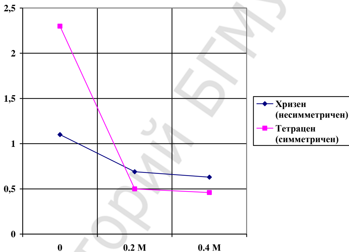
Рис. 1 – Зависимость константы распределения углеводорода от симметричности строения углеводорода
