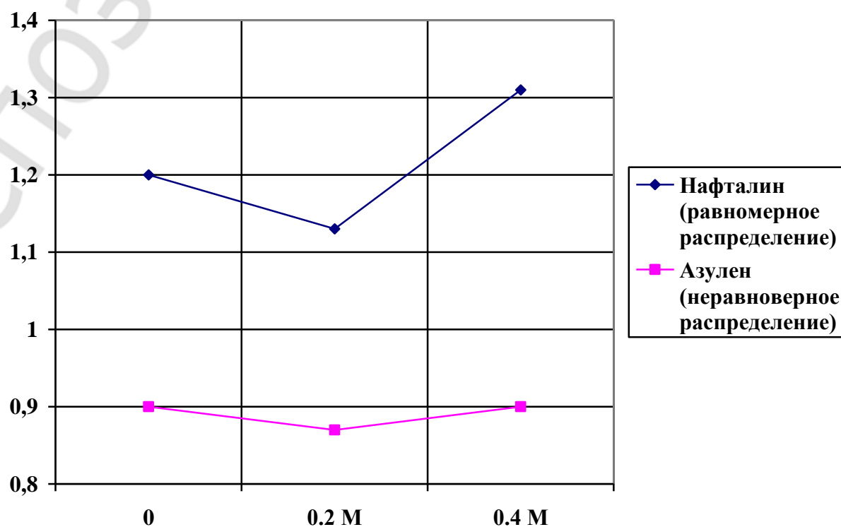
Рис. 1 – Зависимость константы распределения углеводорода от симметричности строения углеводорода
