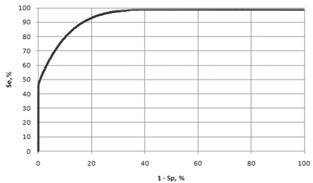
Рис.5. ROC-кривая оценки эффективности прогнозно-диагностической модели
