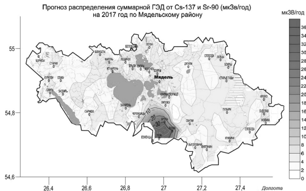
Рис. 1. Прогноз распределения ГЭД (в мкЗв/год) за счет Cs^{137} и Sr^{90} на территории Мядельского района Минской области на 2017 год (по оси абсцисс – градусы восточной долготы, по оси ординат – градусы северной широты)
