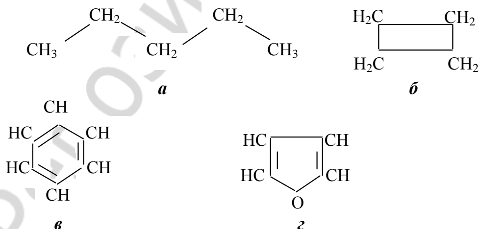
Рис. 2. Представители различных классов органических соединений: а — ациклическое (н-пентан); б — алициклическое (циклобутан); в — ароматическое (бензол); г — гетероциклическое (фуран)
