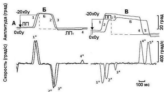
Рис.2. Электроокулограммы саккадических движений глаз. А (сверху) - световая стимуляция. Сплошной линией изображено положение видимой точечной цели на экране и ее координаты по осям X и Y. В момент отмеченный стрелкой цель мгновенно смещается с центра экрана (координата 0x0y) на 20 град влево (в координату -20x0y) и остается там в течение 300 мс. Штриховой линией показан промежуток времени 300 мс, в течение которого цель на экране отсутствовала до ее появления в центре экрана. Б (сверху): 1 - нормометричные ЦФС влево, 2 - нормометричная ЦФС, 3 - ошибочная гиперметричная ЦФС, 4 - коррекционная саккада. В (сверху): 1 - нормометричная ЦФС, 2 - ошибочная гипометричная ЦФС, 3 - коррекционная саккада, 4,5 - нормометричные ЦФС. ЛП, ЛП1, ЛП2 - латентные периоды саккад, 6 - межсаккадический период фиксации взгляда. Б, В (снизу): графики изменения угловых скоростей глаз 1*, 2*, 3*, 4*, 5* во время осуществления саккад 1,2,3,4,5, соответственно.
