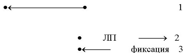
Рис.3. Схематическое представление левостороннего смещения визуальной цели (•) на экране монитора (1), нормальной антисаккады глаз в мнимую точку через латентный период - ЛП (2), периода фиксации и ЦФС (3).
