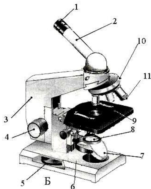
Рис. 1. Устройство светового микроскопа БИОЛАМ:
