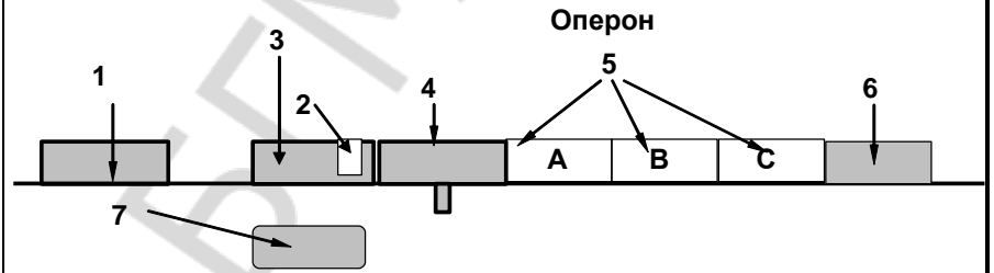
Рис. 1. Схема строения оперона
