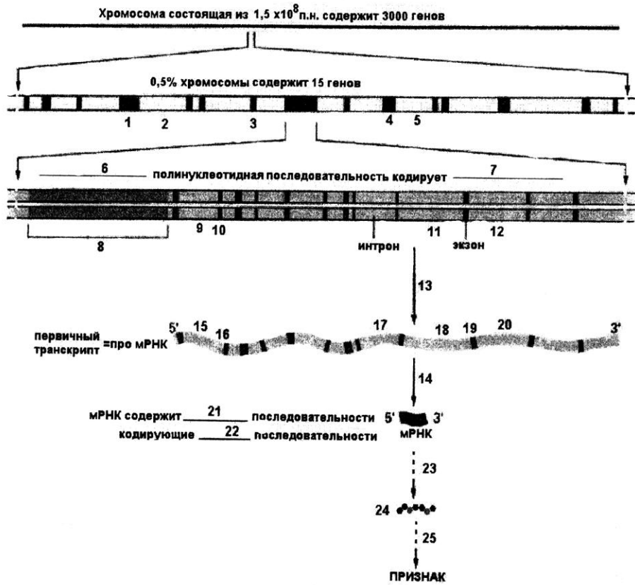
Схема строения и экспрессии генов
