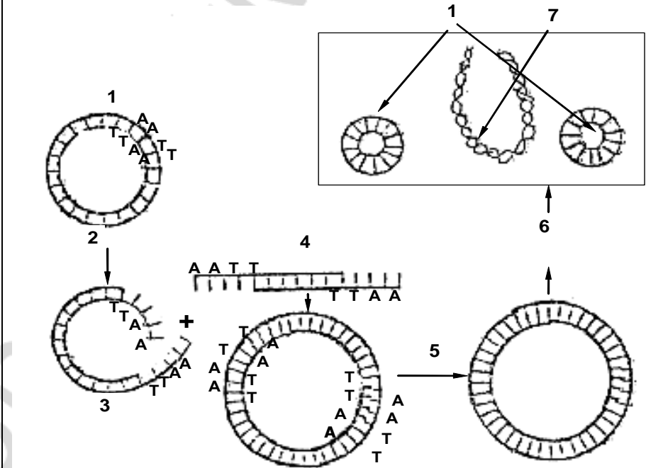
Рис. 1. Схема встраивания гена в плазмиду и введения рекомбинантной плазмиды в бактерию
