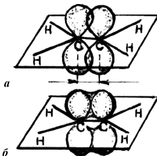
Рис. 7. Схема образования \pi -связи в молекуле этилена: а — боковое перекрытие облаков р-электронов; б — распределение общего облака \pi -связи над плоскостью и под плоскостью атомных ядер
