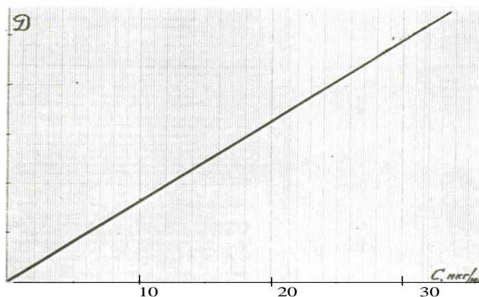
Калибровочный график зависимости величины оптической плотности раствора (D) от концентрации ПВК в пробе
