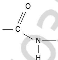
Пептидная связь
