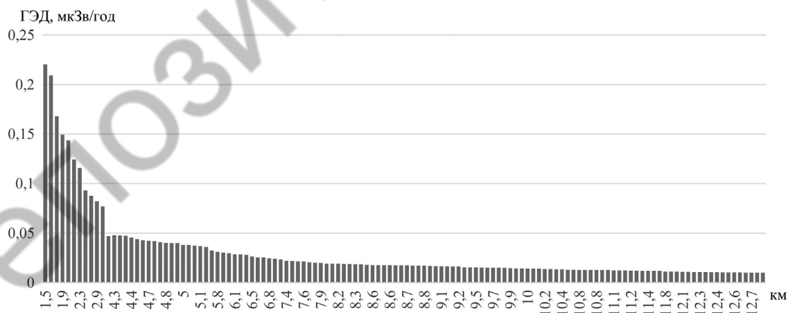
Рисунок 4. Дозы внутреннего облучения за счет перорального поступления ^{131}\text{I} в населенных пунктах, расположенных в зоне наблюдения БелаЭС (мкЗв/год)
