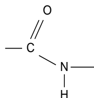
Пептидная связь
