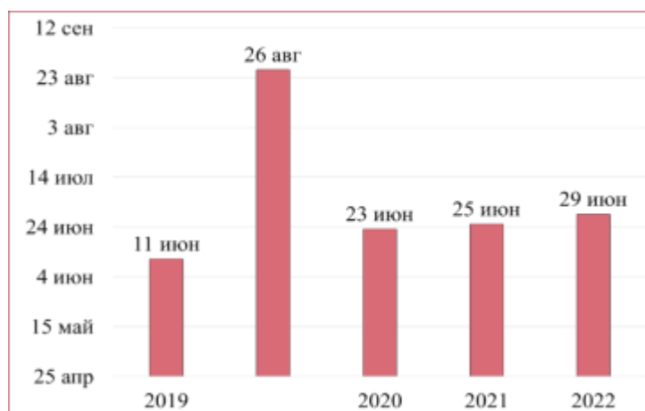
Рис. 3 – Даты начала сезона передачи малярии
