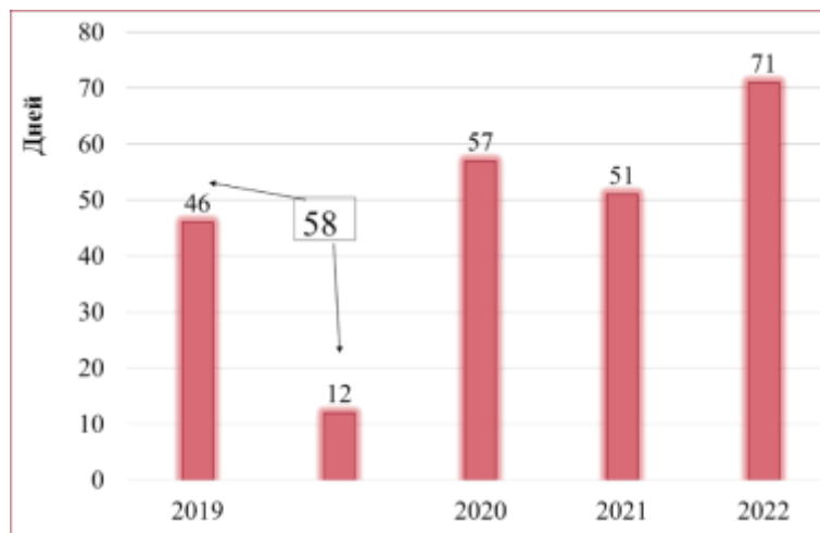
Рис. 2 – Длительность сезона эффективной заражаемости комаров
