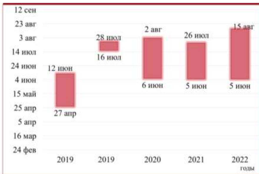
Рис. 1 – Даты начала и окончания сезона эффективной заражаемости комаров
