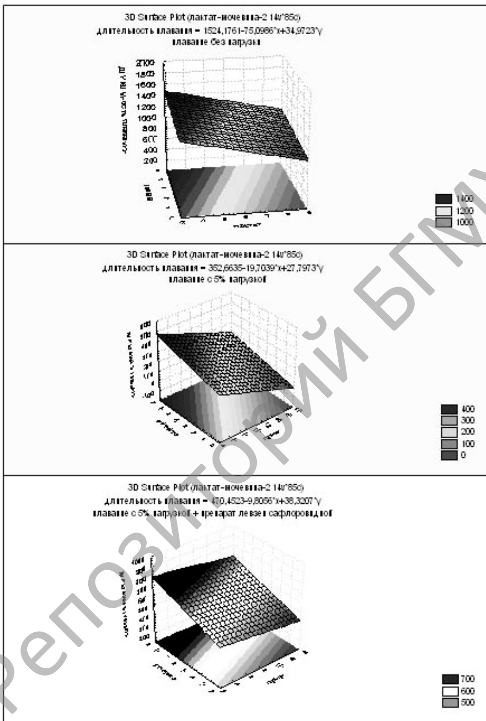
Рисунок 4 Сопряженные показатели длительности плавания и содержания лактата и мочевины в различных группах наблюдения
