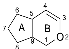
Циклопентанопиран
