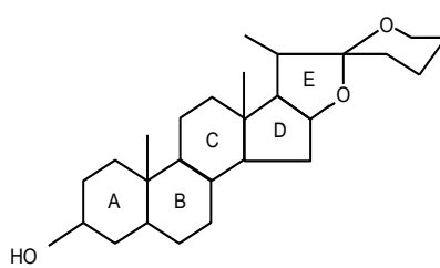
Стероидный сапонин спиростанолового типа
