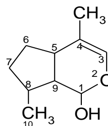
Иридоидиаль (лактонная форма)
