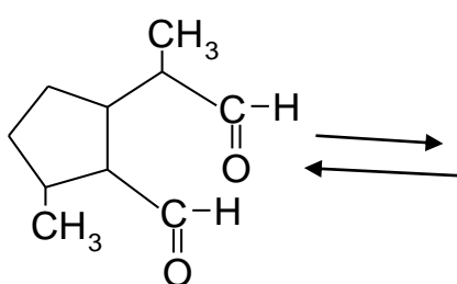
Иридоидиаль (диальдегидная форма)
