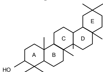
Тритерпеновый сапонин типа \alpha -амирина
