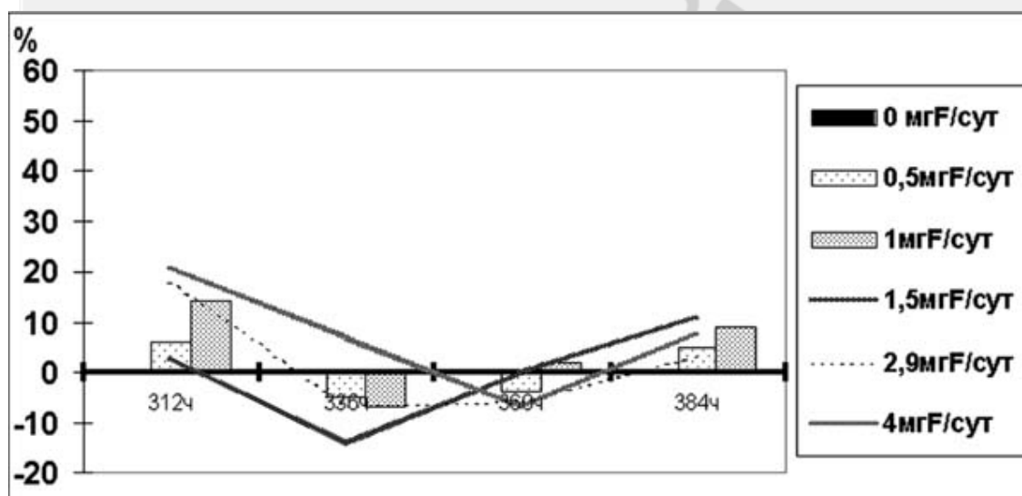
Рис 2. Изменения динамики развития популяций инфузорий Tetrahymena pyriformis в течение седьмого жизненного цикла в условиях, соответствующих фторнагрузке взрослого человека в диапазоне от 0 до 4 мгF/сутки.
