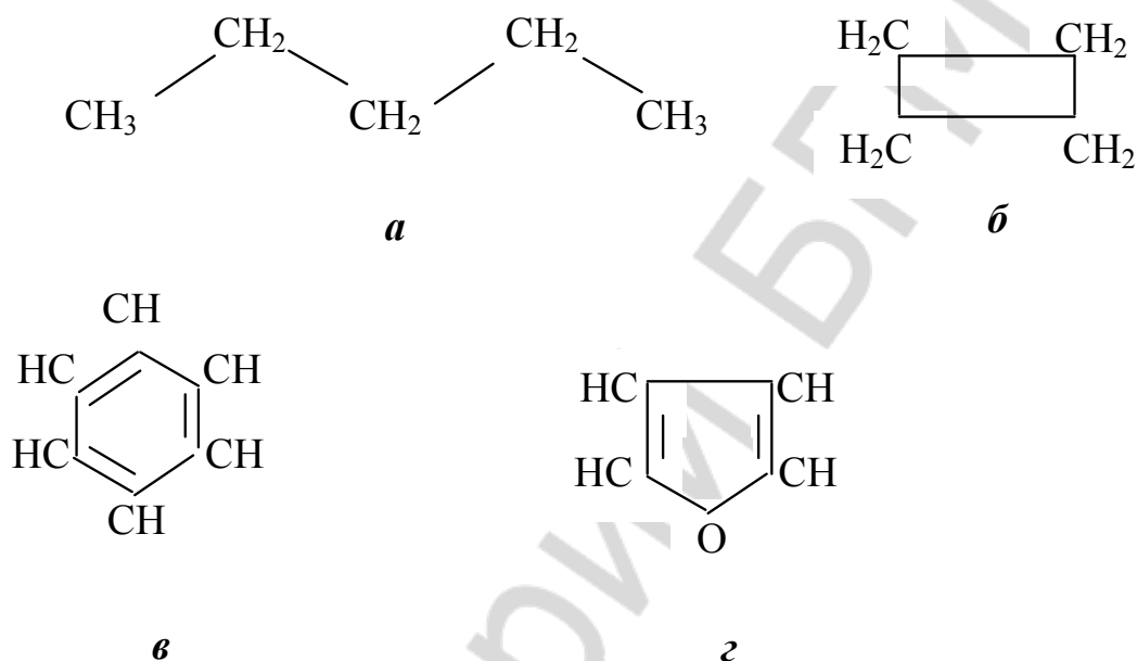
Рис. 1. Представители различных классов органических соединений: a — ациклическое (н-пентан); б — алициклическое (циклобутан); в — ароматическое (бензол); г — гетероциклическое (фуран)
