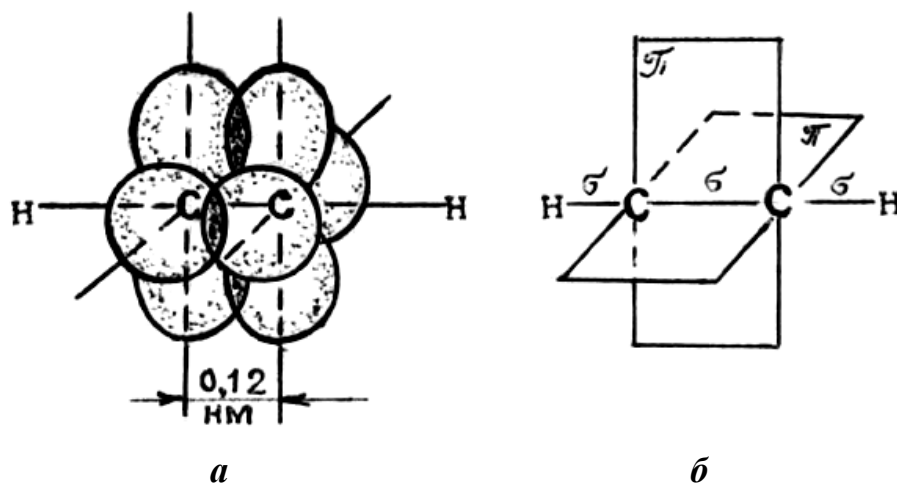
Рис. 7. Схема образования \pi -связей в молекуле ацетилена:
