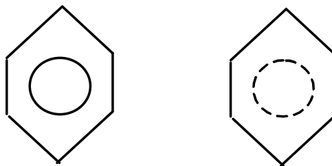
Рис. 8. Схема образования \sigma -связей в молекуле бензола
