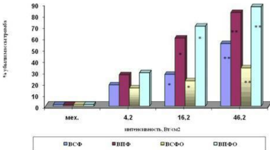
Рисунок 1 - Влияние интенсивности УЗ на степень убыли тромба в зависимости от конструкции головки волновода
