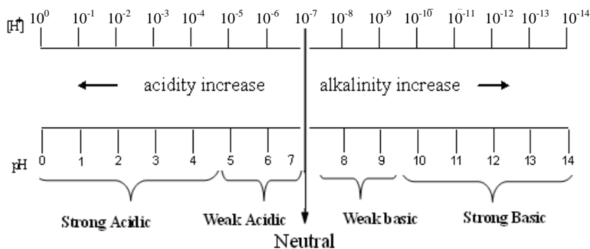
Fig. 6.1. pH scale
