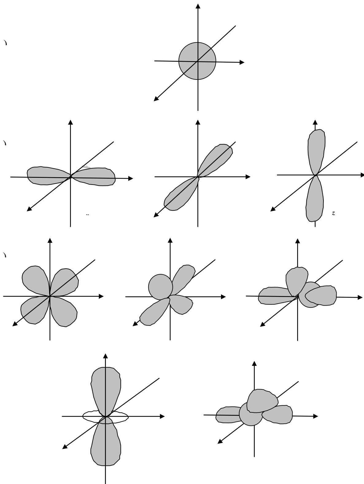
Рис. 2. Формы и пространственная ориентация атомных орбиталей: a — s -орбиталь; b — p -орбиталь; v — d -орбиталь
