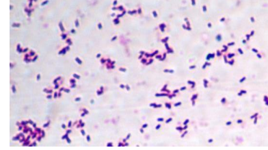
L. monocytogenes
