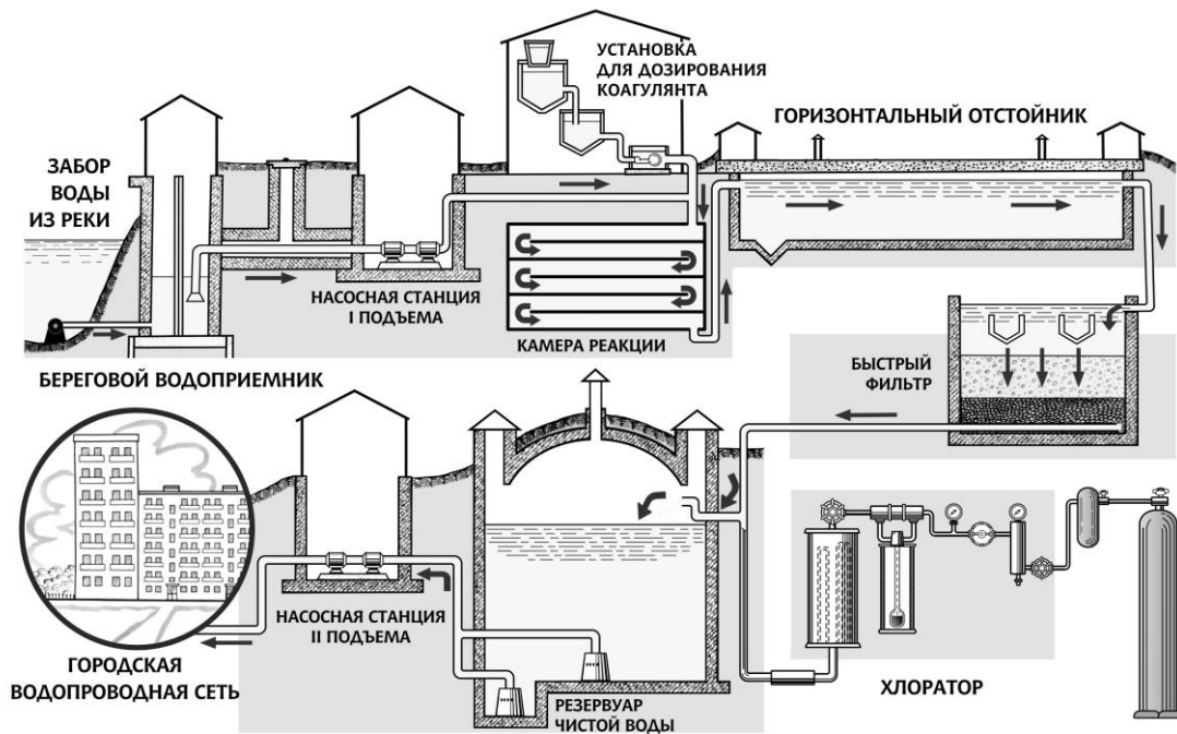
Рис. 2. Схема водопровода из поверхностного источника
