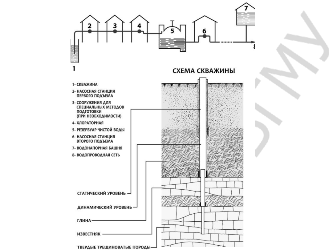
Рис. 1. Схема водопровода из подземного источника
