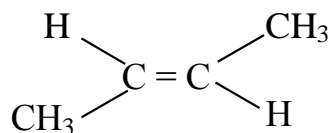
транс-бутен-2
