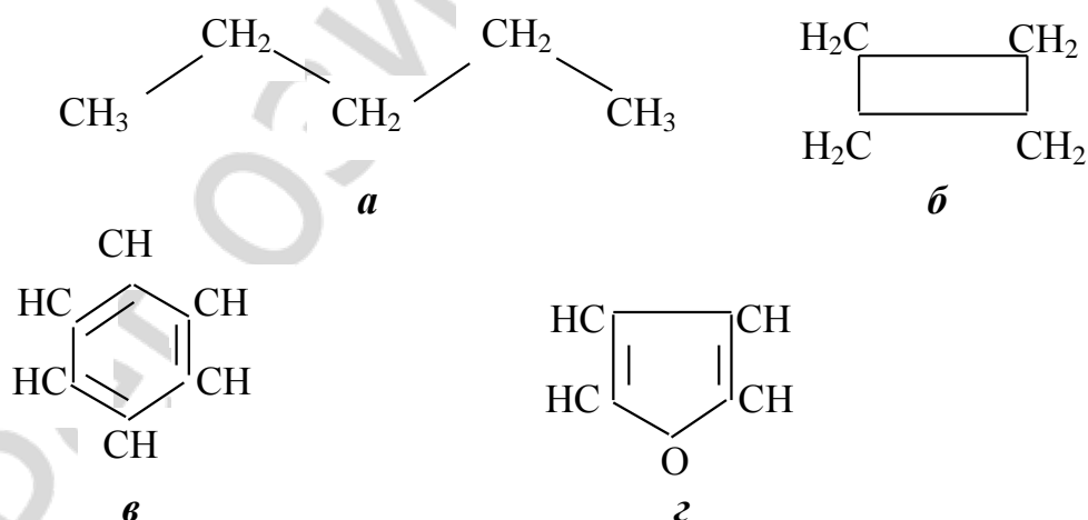
Рис. 2. Представители различных классов органических соединений: а — алициклическое (н-пентан); б — алициклическое (циклобутан); в — ароматическое (бензол); г — гетероциклическое (фуран)
