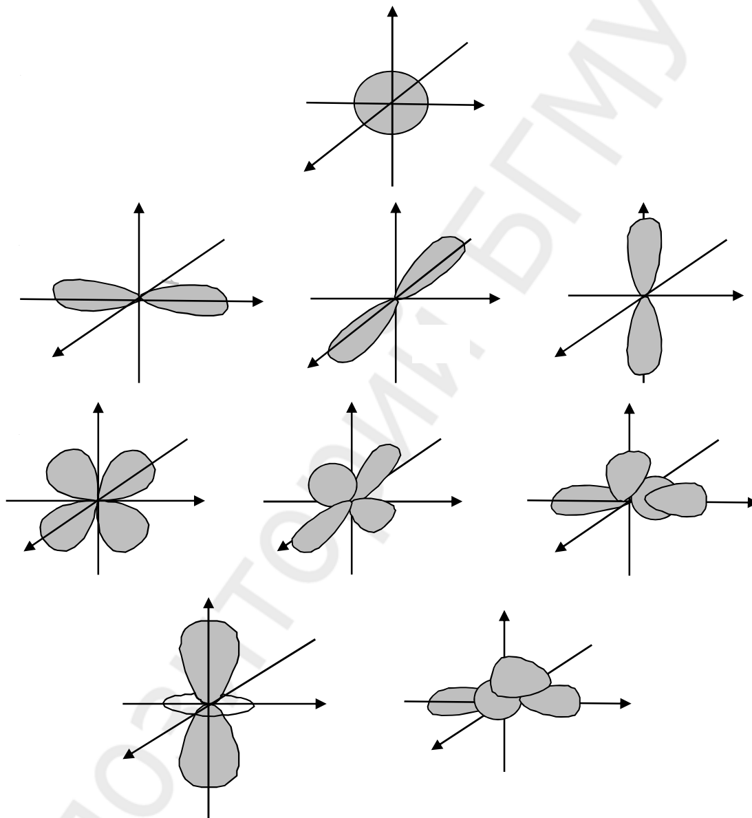
а — s-орбиталь; б — p-орбиталь; в — d-орбиталь
