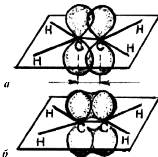
Рис. 7. Схема образования \pi -связи в молекуле этилена: а — боковое перекрывание облаков р-электронов; б — распределение общего облака \pi -связи над плоскостью и под плоскостью атомных ядер
