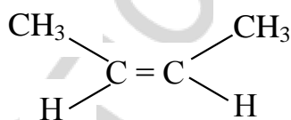
цис-бутен-2
