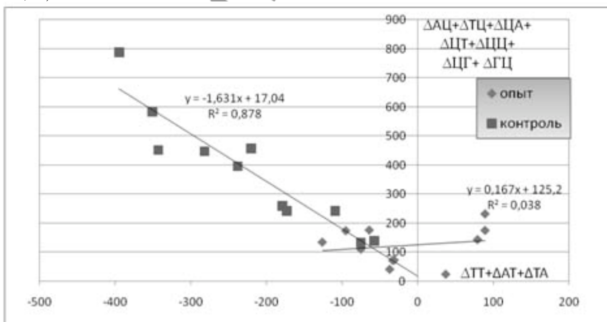
Рисунок 2. Зависимость разницы содержания динуклеотидов АЦ+ТЦ+ЦА+ЦТ+ЦЦ+ЦГ+ГЦ от разницы содержания динуклеотидов ТТ+АТ+ТА в
