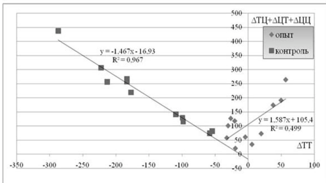
Рисунок 1. Зависимость разницы содержания динуклеотидов ТЦ+ЦТ+ЦЦ от разницы содержания динуклеотидов ТТ в сравниваемых ДНК человека и трихинеллы (опыт), человека и цианорабдитис (контроль).
