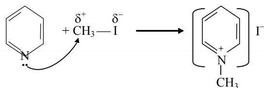
йодид N-метилпиридиния
