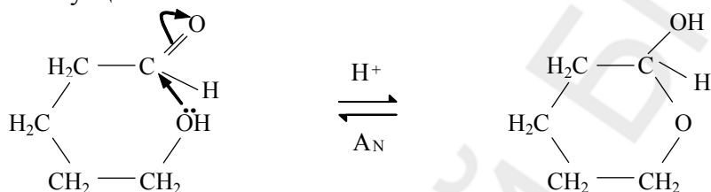
5-гидроксипентаналь
