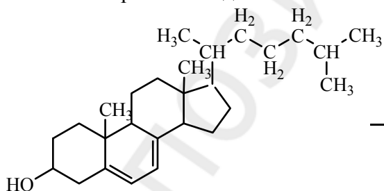
7-дегидрохолестерол
