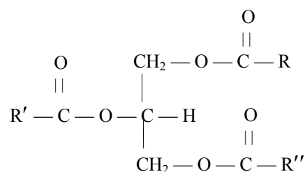
триацилглицерол
