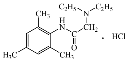
тримекаина гидрохлорид
