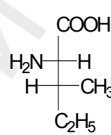
L-алло-изолейцин
