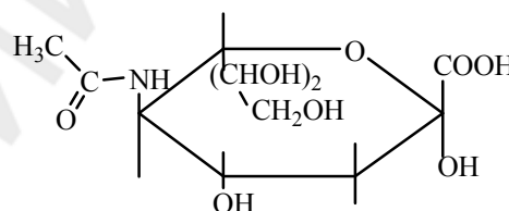
N-ацетилнейраминовая кислота
