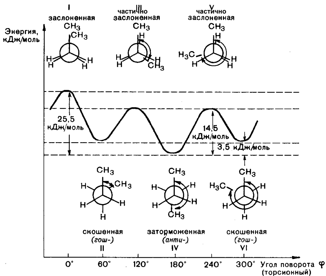
Потенциальная энергия конформаций н-бутана
