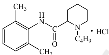
бупивакаина гидрохлорид
