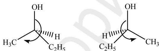
R-изомер
