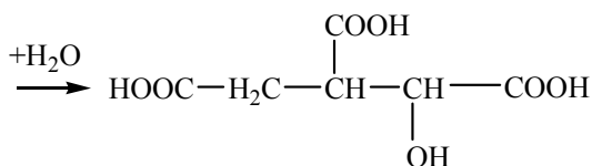
изолимонная кислота
