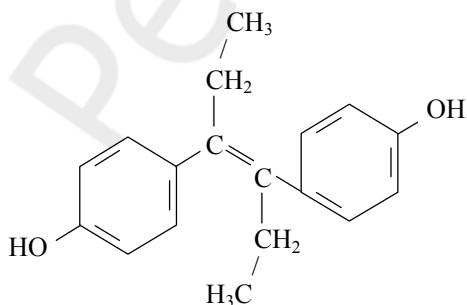
диэтилстильбэстрол
