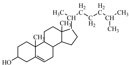
холестерол
