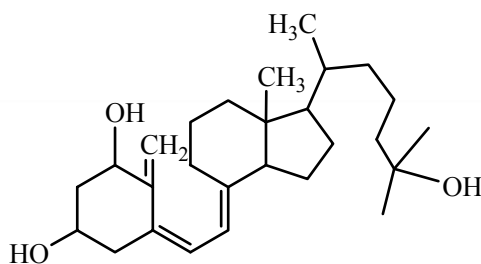
1,25-дигидроксиголекальциферол
