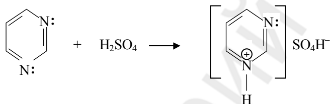
пиримидиний гидросульфат
