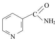
никотинамид
