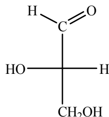
(-) L-глицериновый альдегид
