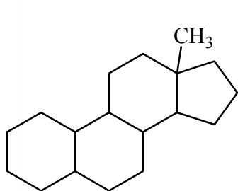
ýñòðàí
