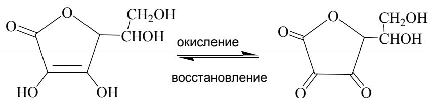
окисленная форма
