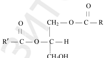
1,2-диацилглицерол
