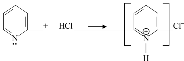
хлорид пиридиния
