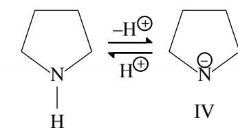
пирролидин
