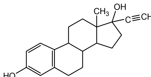
этинилэстрадиол
