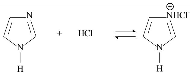
имидазола гидрохлорид
