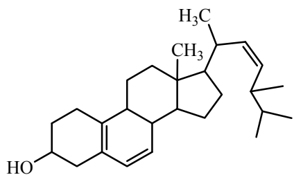
эргостерин
