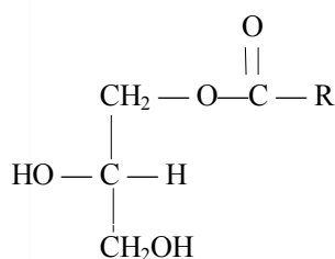
моноацилглицерол
