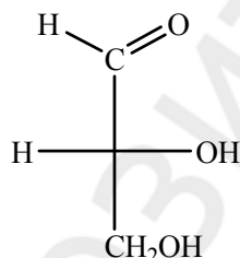
(+) D-глицериновый альдегид
