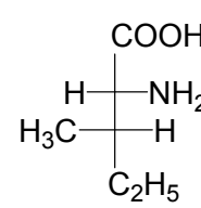
D-алло-изолейцин
