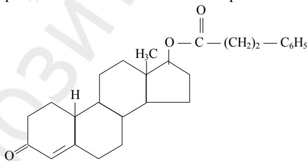
нероболит
