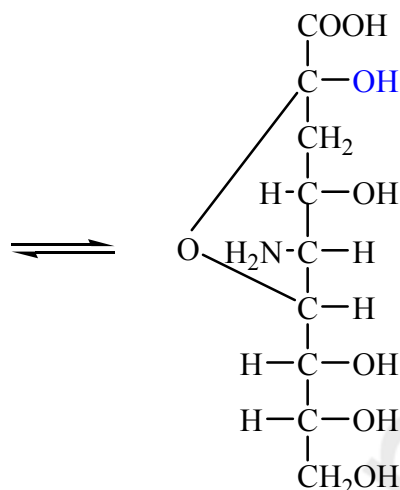
нейраминовая кислота
