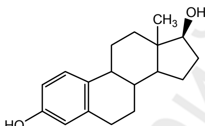
ýñòðàäèë ì-17β
