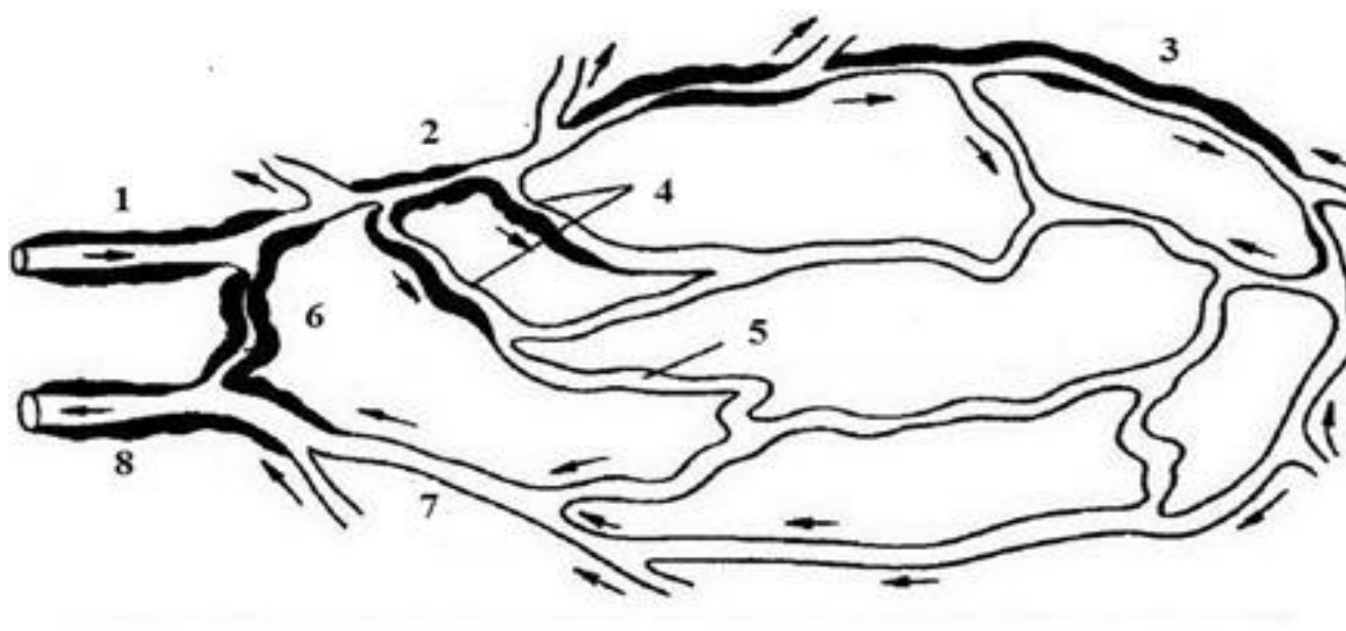
Рис. 3. Принципиальная схема микроциркуляции (по В. В. Zweifach)
