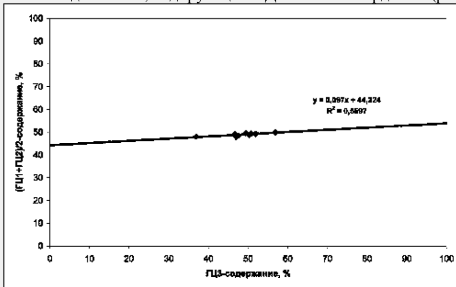
Рис. 2. Зависимость между (GC1+GC2)/2 -содержанием и GC3-насыщенностью мРНК, кодирующих АДГ класса 1 хордовых животных. Наклон тренда для мРНК, кодирующих АДГ1, составляет 0,097, а значит нейтральность замен равна 9,7% и степень селективных ограничений составляет 90,3%.
