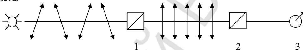
Схема поляриметра:
