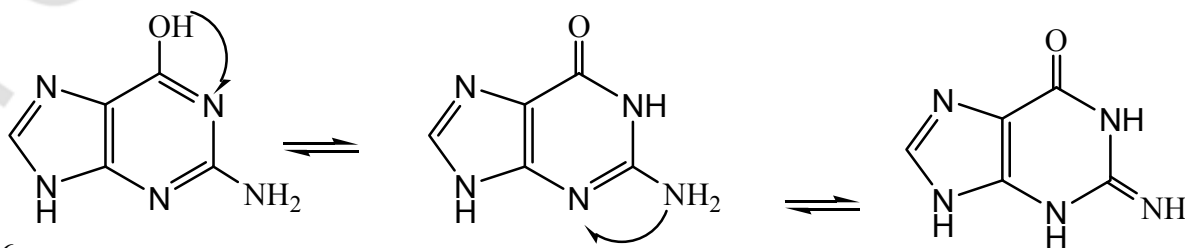
лактамная форма аминная форма
