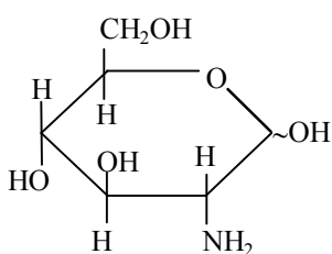
D-глюкозамин
