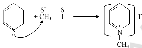
йодид N-метилпиридиния
