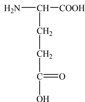
2-аминопентандиовая кислота L-глутаминовая кислота Glu
