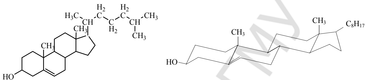
холестерол
