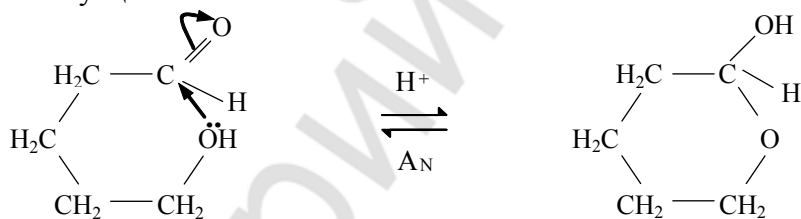
5-гидроксипентаналь
