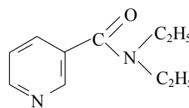
кордиамин
