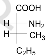
D-изолейцин
