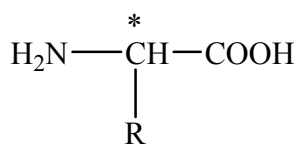
\alpha -аминокислота
