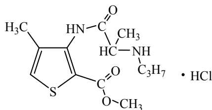
ультракаина гидрохлорид
