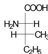
L-алло-изолейцин
