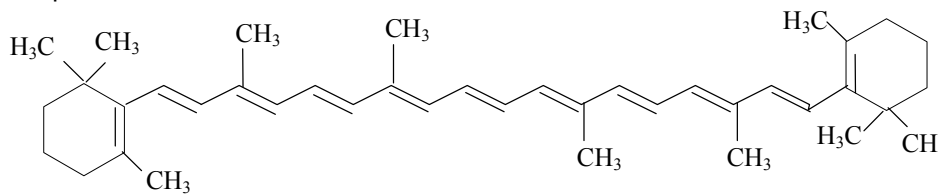
\beta -каротин
