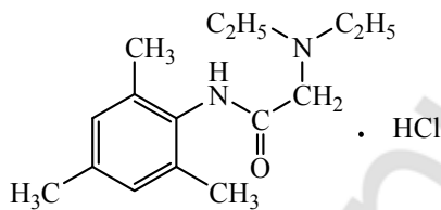
тримекаина гидрохлорид
