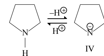
пирролидин
