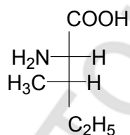
L-изолейцин
