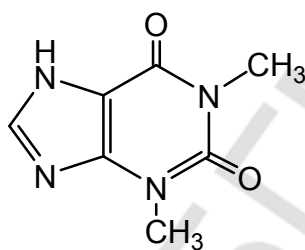
теofilлин 1,3-диметилксантин
