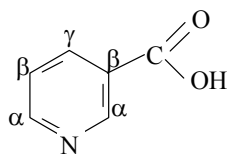
никотиновая кислота
