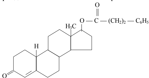
нероболлил
