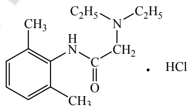
лидокаина гидрохлорид
