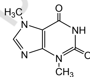
теобромин 3,7-диметилксантин
