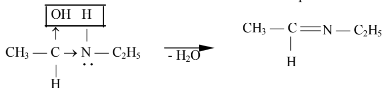
N-замещенный имин
