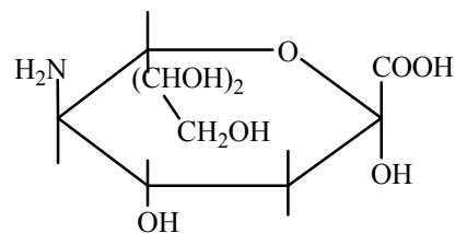
нейраминовая кислота по Хеурсу
