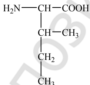
2-амино-4-метилпентановая кислота
