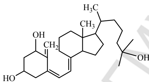
1,25-дигидроксихолекальциферол
