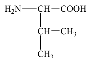
2-амино-3-метилбутановая кислота L-валин Val
