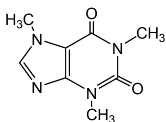
кофеин 1,3,7-триметилксантин
