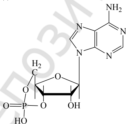
аденозин-3',5'-циклофосфат 3',5'-циклоАМФ
