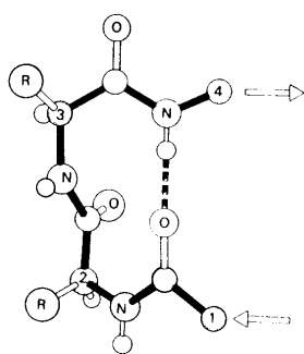
\beta -Изгиб.
