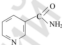
никотинамид
