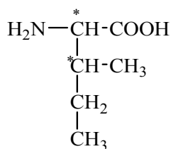
изолейцин
