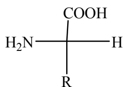
L- \alpha -аминокислота
