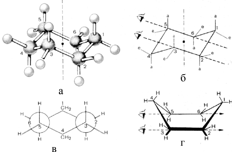
Конформации циклогексана:
