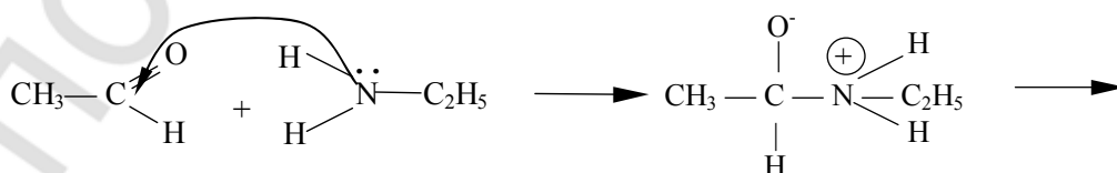
биполярный ион
