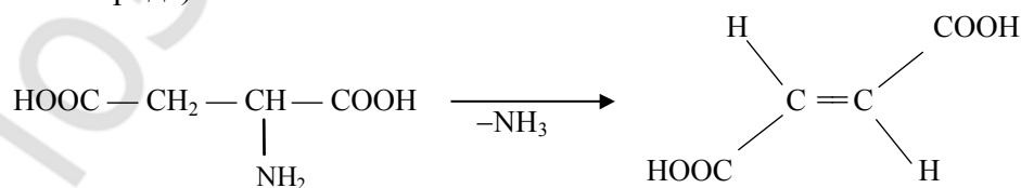
аспарагиновая кислота
