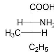
D-алло-изолейцин
