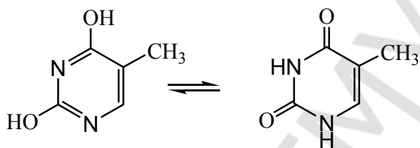
2,4-дигидрокси-5-метилпиримидин лактимная форма лактамная форма
