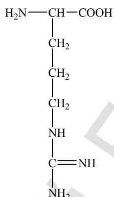
2-амино-5-гуанидилпентановая кислота L-аргинин Arg
