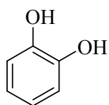
пирокатехин катехол
