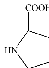
2-пирролидин-карбоновая кислота L-пролин Pro
