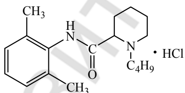
бупивакаина гидрохлорид
