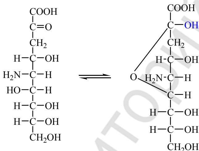
нейраминовая кислота
