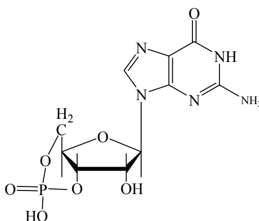
гуанозин-3',5'-циклофосфат 3',5'-циклоГМФ
