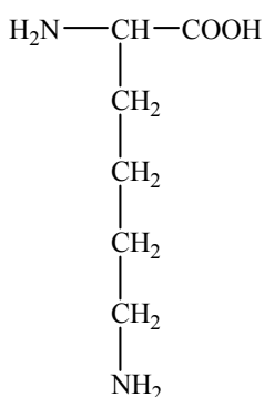
2,6-диаминогексановая кислота L-лизин Lys
