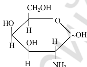
D-галактозамин
