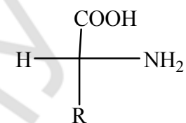
D- \alpha -аминокислота
