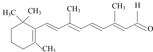
ретиаль
