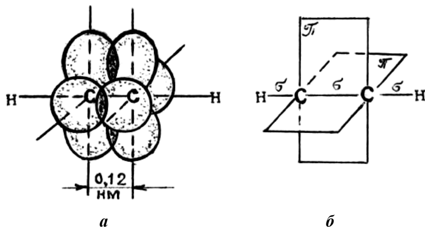
Рис. 7. Схема образования \pi -связей в молекуле ацетилена:
