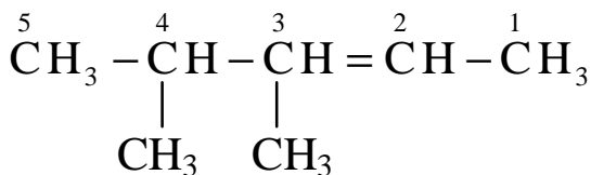
3,4 диметилпентен-2
