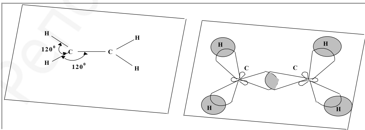
Рис. 5. Схема образования \sigma -связей в молекуле этилена
