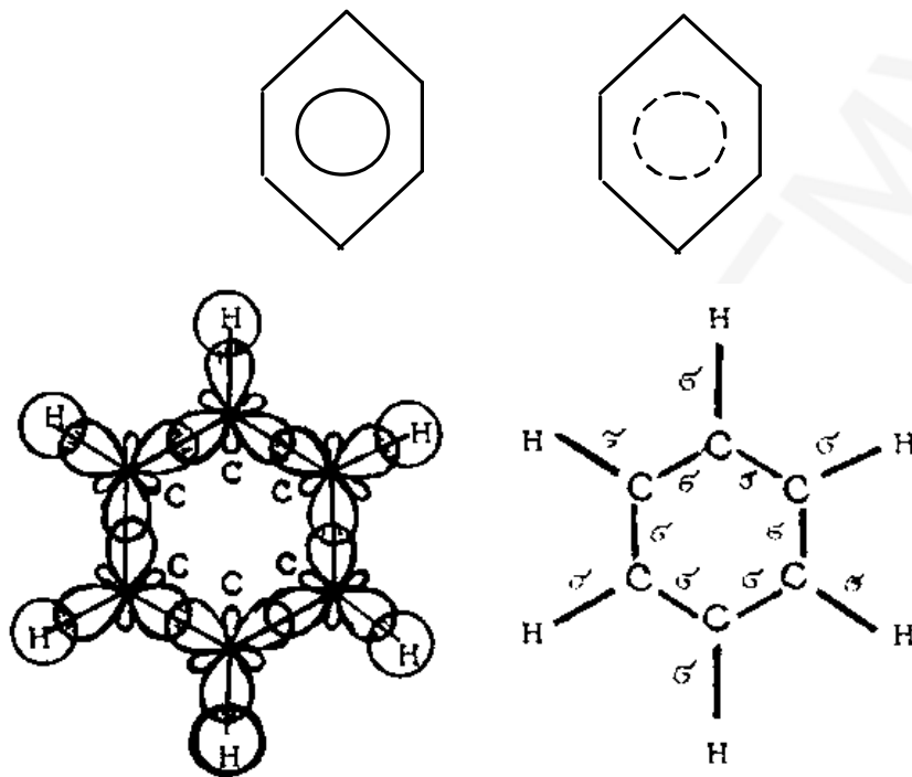
Рис. 8. Схема образования \sigma -связей в молекуле бензола
