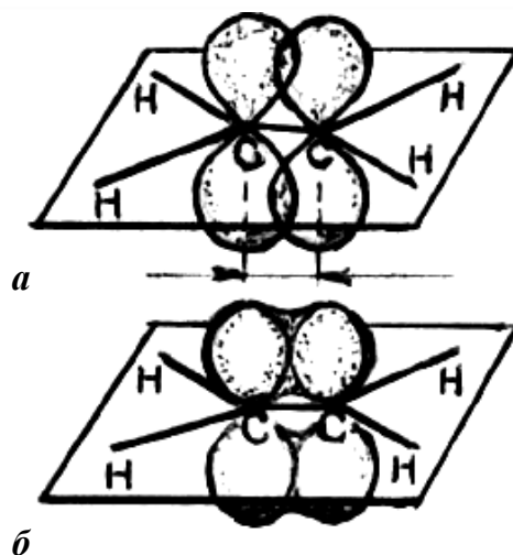
Рис. 6. Схема образования \pi -связи в молекуле этилена: а — боковое перекрывание облаков р-электронов; б — распределение общего облака \pi -связи над плоскостью и под плоскостью атомных ядер
