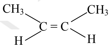
цис-бутен-2
