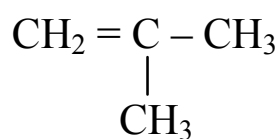
2-метил-пропен-1
