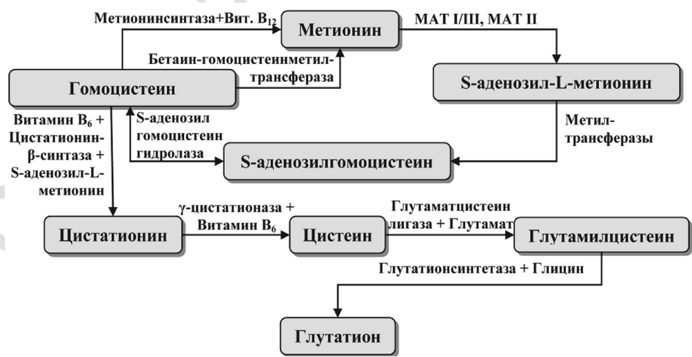
Рис. 2. Участие адеметионина в синтезе глутатиона
