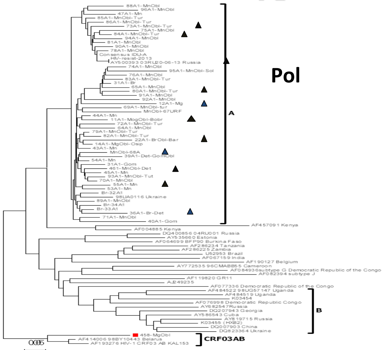
Рисунок 1 - Филогенетическое дерево, построенное в результате секвенирования по гену pol
