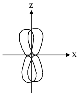
Рис. 4. Образование π-связи
