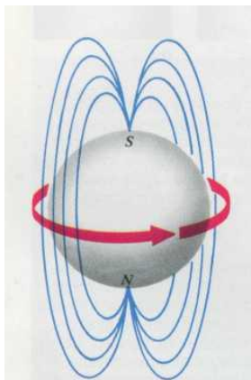
Fig. 1.5. Electron spin
