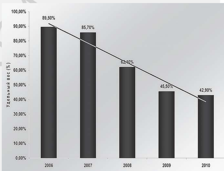
Рисунок 3 Динамика удельного веса штаммов Haemophilus influenzae типа b чувствительных к ко-тримоксазолу за 2006-2010 гг.
