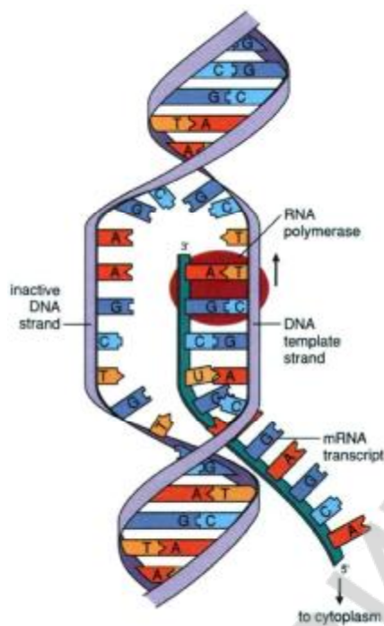
Fig. 17. Transcription
