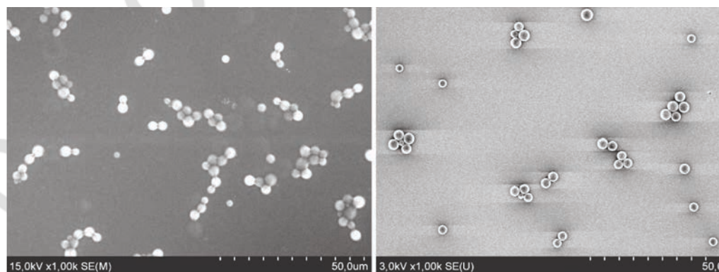
Рисунок 1. СЭМ-изображения ММС а — желатиновые; б — хитозановые
