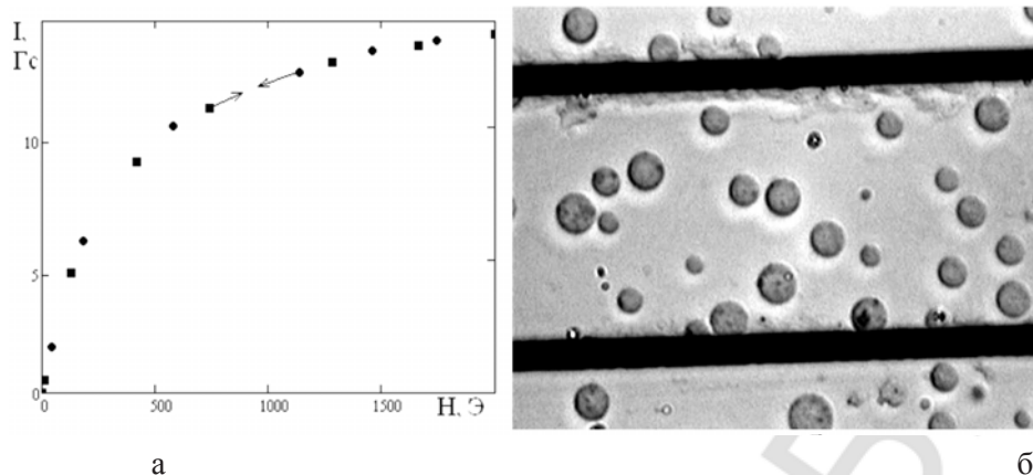
Рисунок 2. Подтверждение суперпарамагнитных свойств ММС а — Кривая намагничивания концентрированного образца суспензии хитозановых ММС при увеличении и уменьшении поля; б — желатиновые ММС в водной среде
