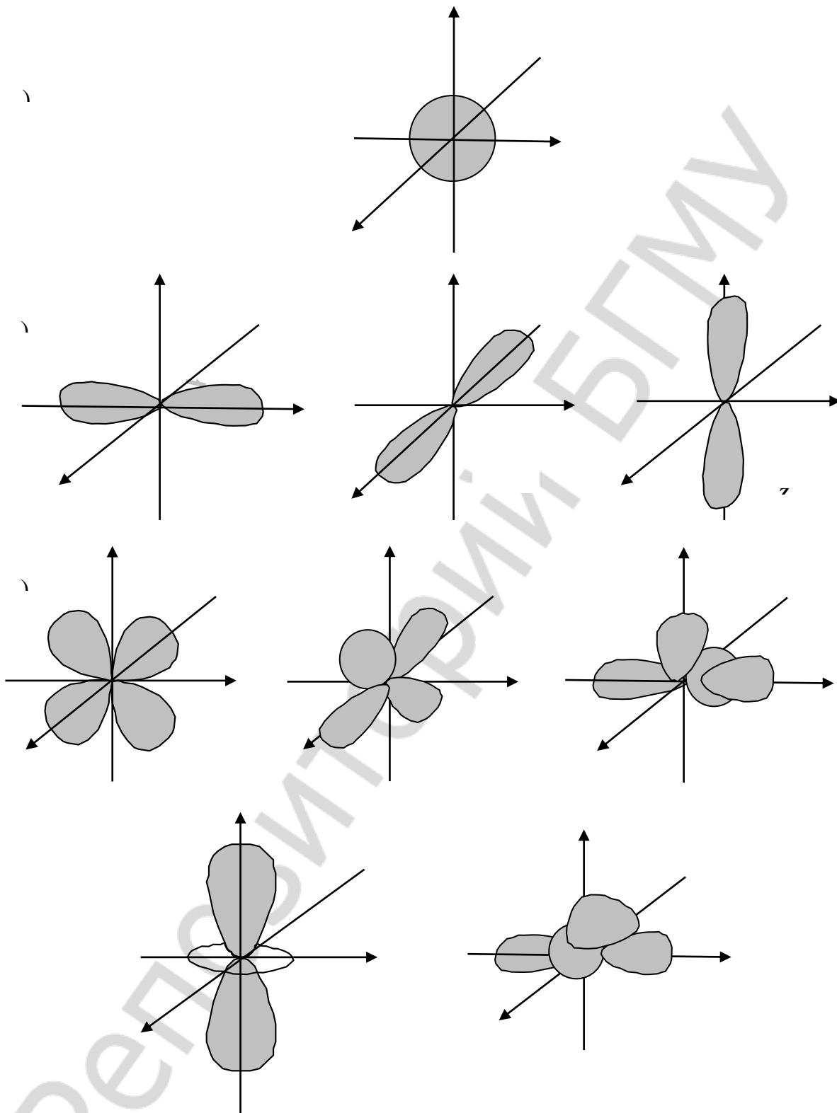
Рис. 2. Формы и пространственная ориентация атомных орбиталей: a — s -орбиталь; б — p -орбиталь; в — d -орбиталь
