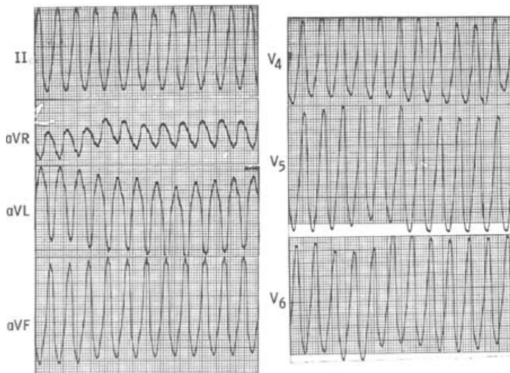
Рис. 5. Трепетание желудочков
