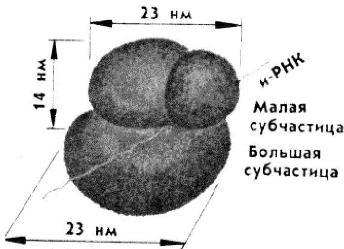
Рис. 68. Строение рибосомы
