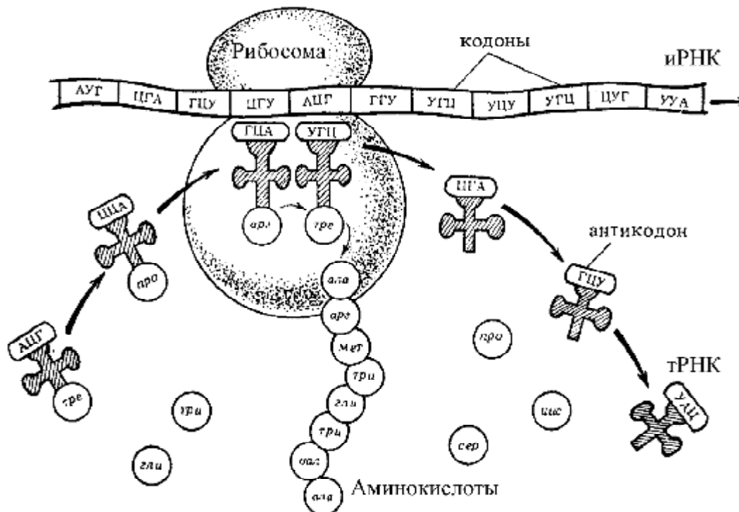
Рис. 75. Трансляция
