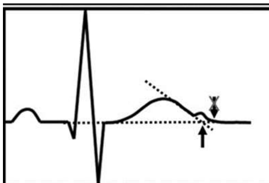
Рис. 2 – Метод «avoid-the-tail»
