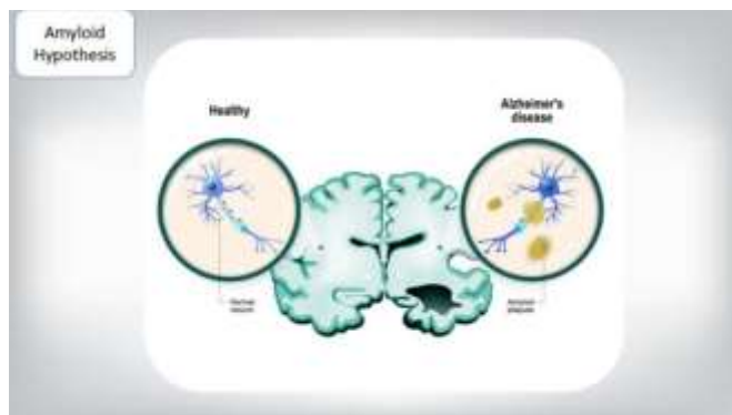
Рис. 1 – Амилоидная гипотеза.
