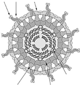
Структура вируса
