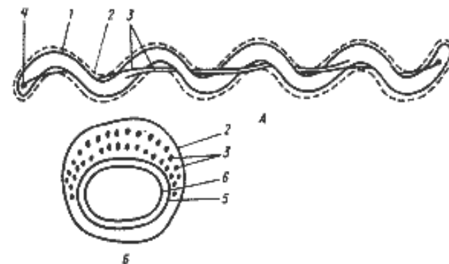
Клетка спирохеты в продольном (А) и поперечном (Б) разрезе. На рис. А изображена клетка, содержащая по одной аксиальной фибрилле у каждого конца; на рис. Б — поперечный разрез, прошедший через среднюю часть клетки, где показаны два пересекающихся пучка, состоящих из множества аксиальных фибрилл: 1 — протоплазматический цилиндр; 2 — наружный чехол; 3 — аксиальные фибриллы; 4 — место прикрепления аксиальных фибрилл; 5 — пептидогликановый слой клеточной стенки; 6 — ЦПМ.
