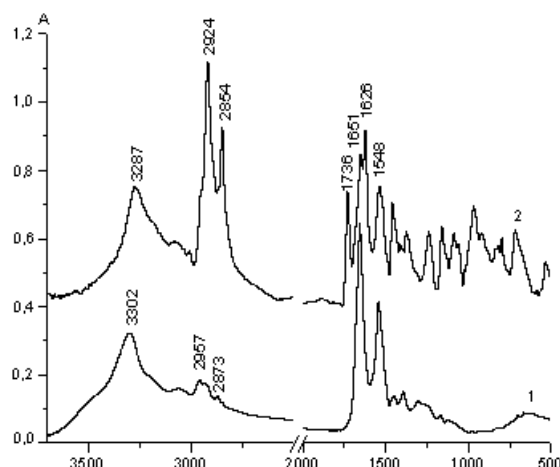
Рис. 1 – ИК-фурье-спектры пленок альбумина (1) и липопротеинов низкой плотности (2) в области частот 500-3600 cm^{-1} (спектры смещены по оси ординат для наглядности)
