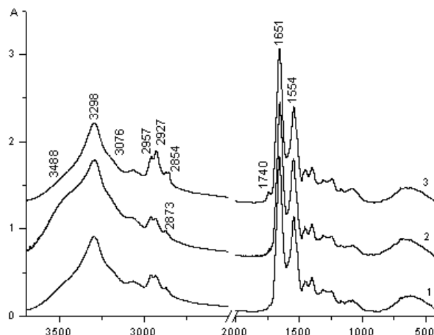
Рис. 2 – ИК-фурье-спектры пленок плазмы крови контрольной группы (1,2) и беременной женщины с Rh-иммунизацией (3) на сроке беременности 30-31 недель в области частот 500\text{--}3600\text{ см}^{-1} (спектры смещены по оси ординат для наглядности)
