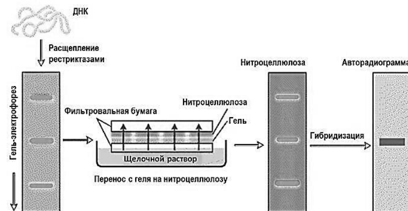
Рис. 3. Саузерн-блоттинг
