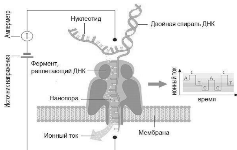
Рис. 2. Нанопоровое секвенирование
