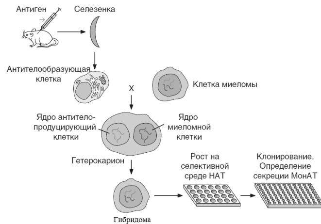
Рис. 2. Технология гибридом
