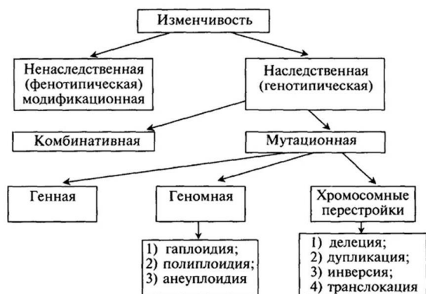
Рис. 1. Виды изменчивости
