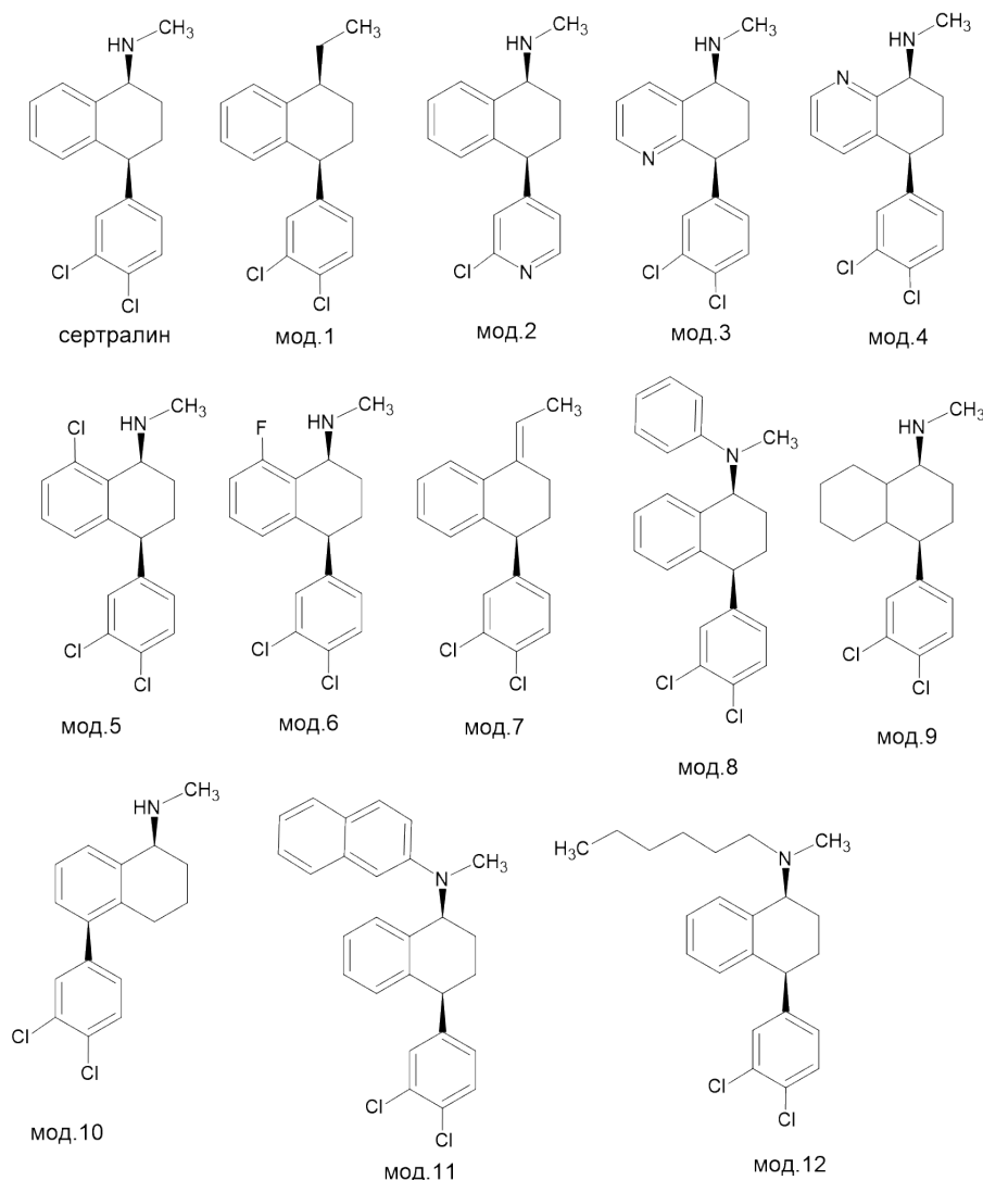
Рис. 3 – Производные Сертралина
