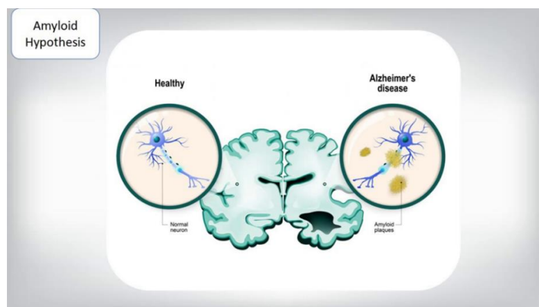
Рис. 1 – Амилоидная гипотеза
