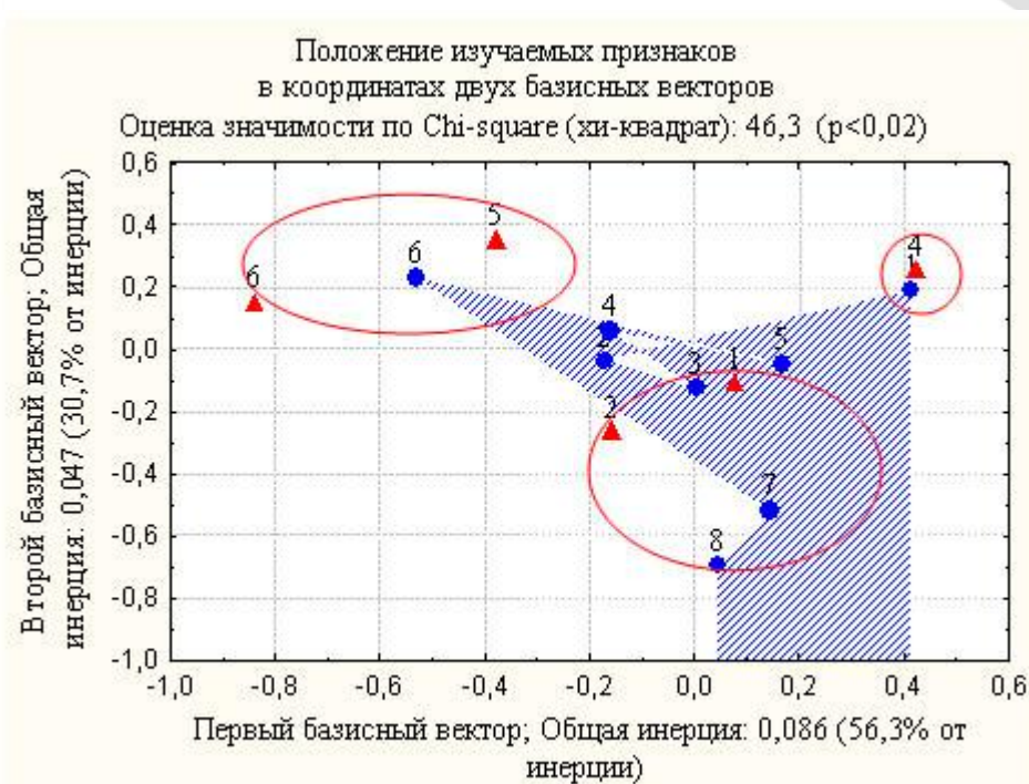
Рис. 1. Диаграмма взаимосвязи по величине инерции (показателю сопряженности \phi ) между ДСиФ и эзофагогастроуденальными заболеваниями
