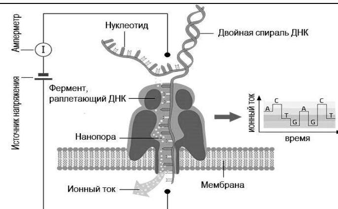
Рис. 6. Нанопоровое секвенирование
