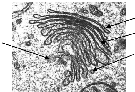
Рис. 6. Электронограмма комплекса Гольджи: 1 — мембрана; 2 — цистерна; 3 — лизосома; 4 — пузырьки
