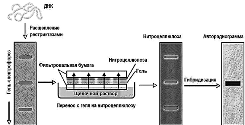
Рис. 3. Саузерн-блоттинг
