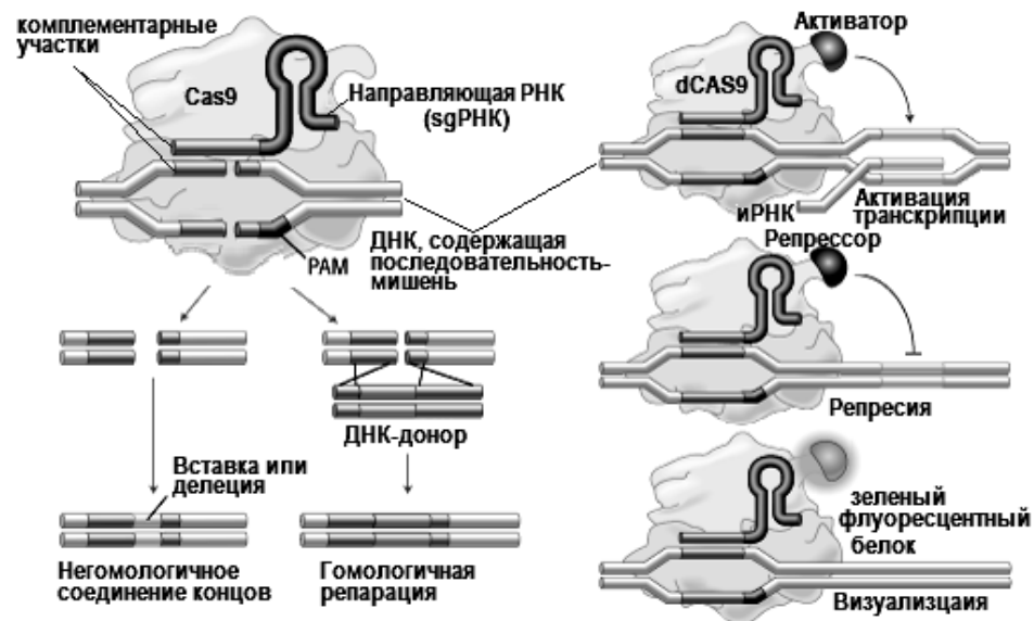
Рис. 4. Применения CRISPR/Cas9
