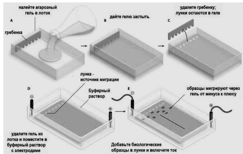
Рис. 2. Гель-электрофорез
